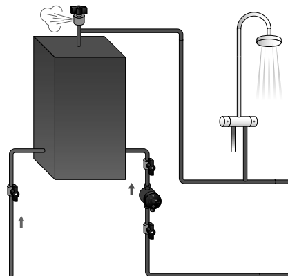
Abb. 5 Häusliches Warmwasserzirkulationssystem
