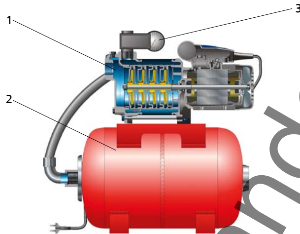
Abb. 4: Schnittbild Multi Eco-Top
