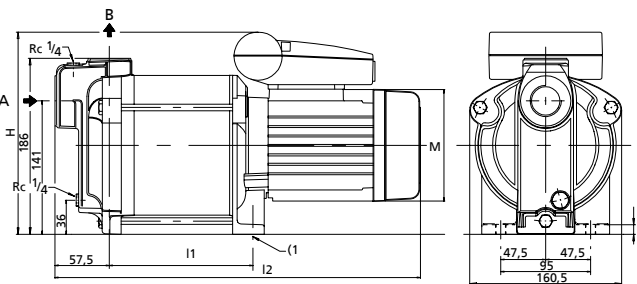
Multi Eco E und D
