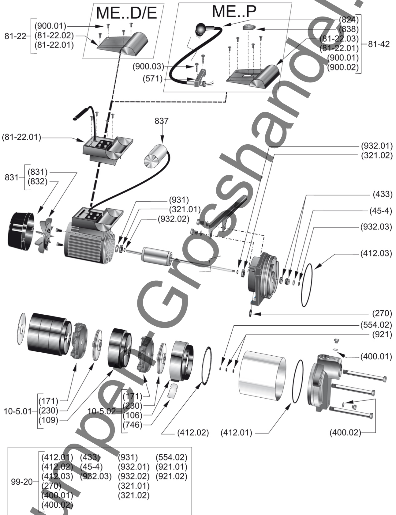
Abb. 5: Explosionsdarstellung
