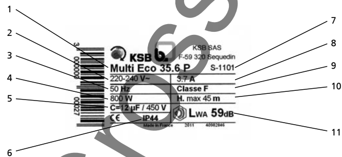
Abb. 1: Typenschild
